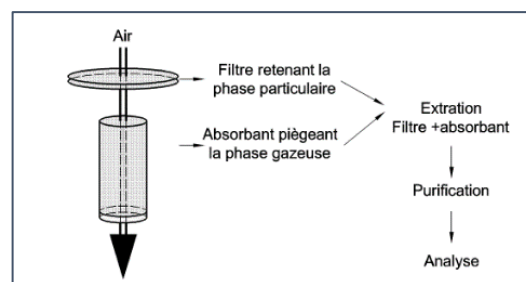
Figure 8 : Dispositif de prélèvement selon la norme XP X43-058
