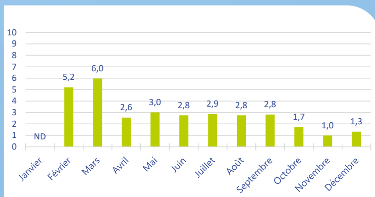
Moyennes mensuelles 2023 pour la surveillance de l'ammoniac sur la station urbaine d'Auxerre (concentrations en \mu\text{g}/\text{m}^3 )
