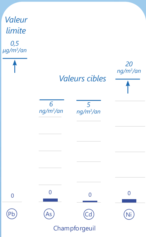
Moyennes 2023 pour la mesure indicative des métaux (en µg/m³ pour le Pb, en ng/m³ pour As, Cd, Ni)
